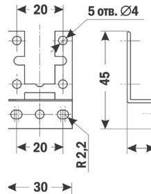
Настенное крепление с помощью комплекта DRM-40-Н.К.
