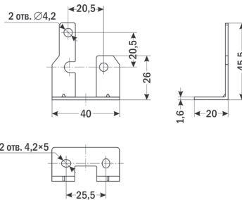
Настенное крепление с помощью комплекта DRM-40-Н.К.
