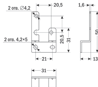
Настенное крепление с помощью комплекта DRM-20-Н.К.
